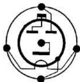
Sockelschaltung
